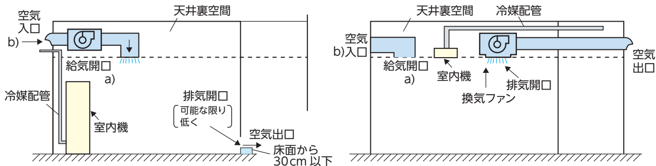
図 16 床置形、天井カセット形室内機の換気装置設置例
